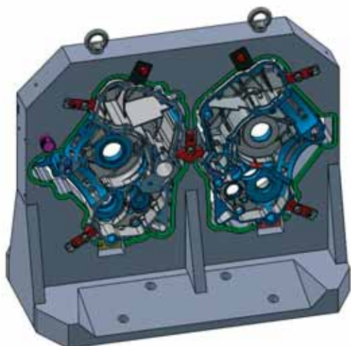
Mechanický upínací přípravek
